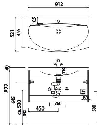
SET VU90
